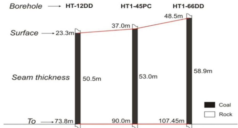
Зураг 4: Үнст худаг төсөл дээр хийсэн өрөмдлөгийн цооног
